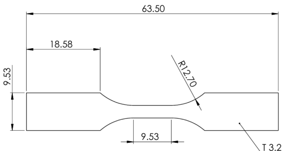
Obr.č.3.1 Rozměry tisknutých vzorků
